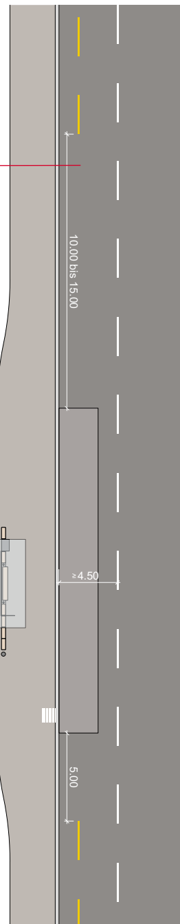
Variante B: Radstreifen wird vor Haltestelle unterbrochen
