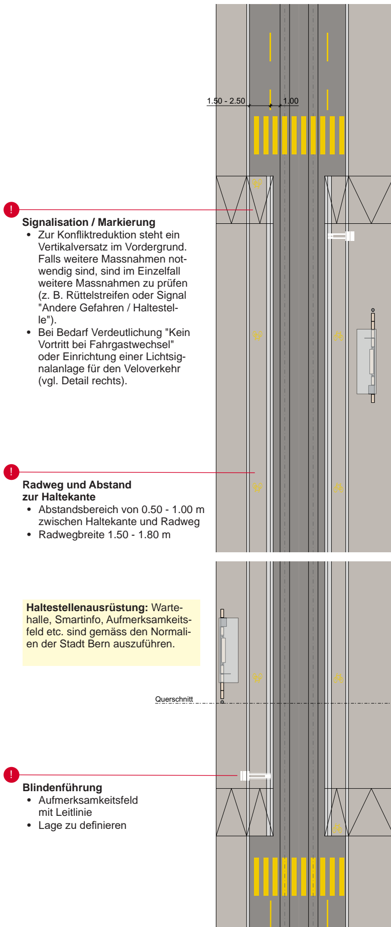
Situationsplan (freier Massstab)
