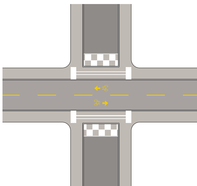
Querung mit Rechtsvortritt und Fussverkehrsquerung.
