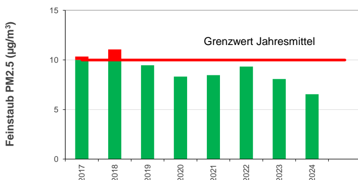
Feinstaub PM2.5-Jahresmittelwerte 2017 - 2024, Bern Morgartenstrasse
