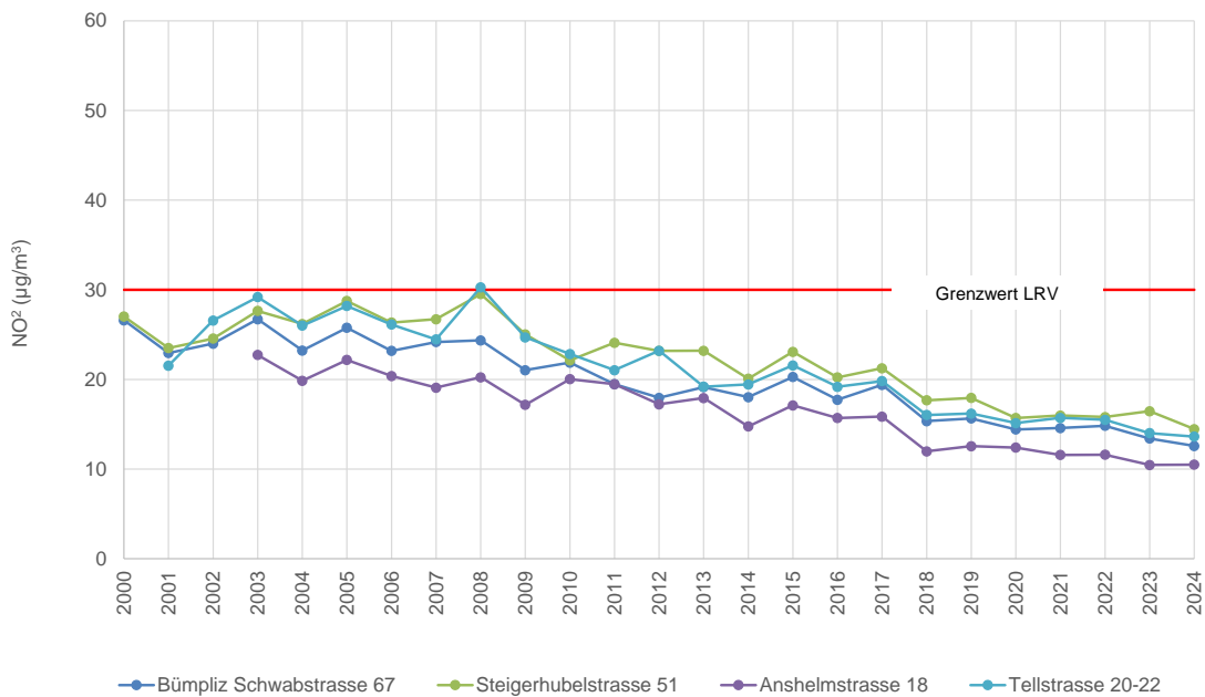
NO 2 -Jahresmittelwerte, Quartierstrassen
