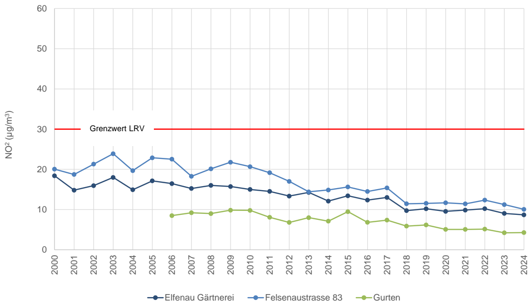
NO 2 -Jahresmittelwerte, ländliche Stationen
