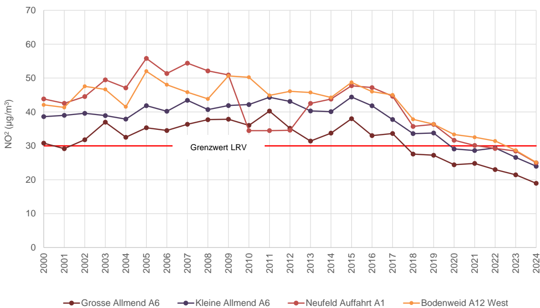
NO 2 -Jahresmittelwerte, Standorte an Autobahnen
