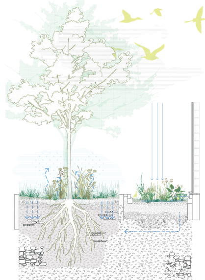
Prinzip Sickerbeet
