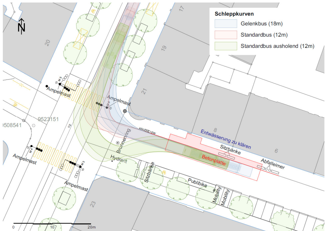
Abbildung 27: Haltekante in Randlage
