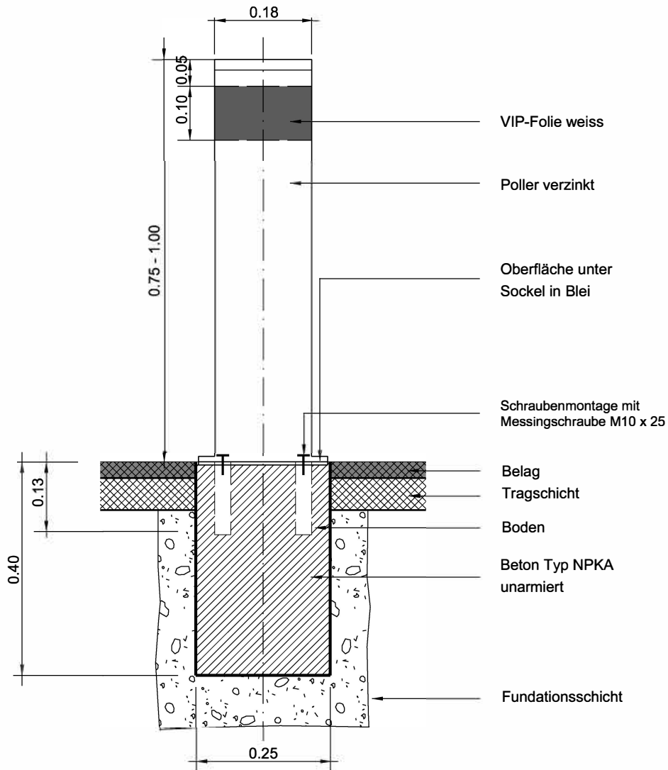
Schnitt A-A mit Betonfundament Masstab 1:10
