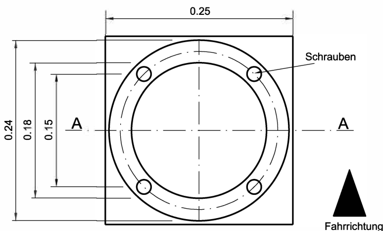
Versetzanordnung Masstab 1:5
