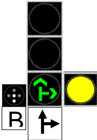
Abbildung 57: Ein Fünf-Punktsignal D = 200 m oben an Mastausleger mit MIV-Signalgeber D = 300 mm.
