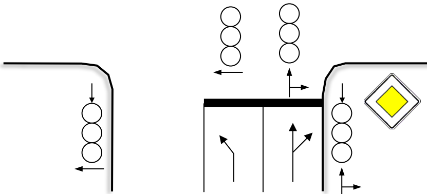
Abbildung 14: Anzahl Signalgeber zwei Fahrstreifen Haupttrichtung ohne Insel.
