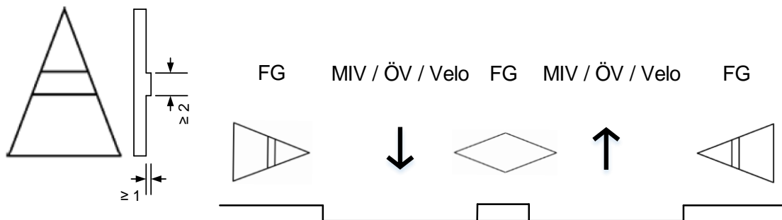
Abbildung 31: Richtungspfeil und Situation «Überweg mit Mittelinsel» [VSS, 2020].
