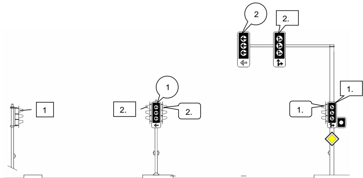
Abbildung 3: Beispiel für Nummerierung der Signalgeber.
