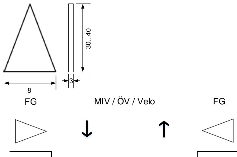
Abbildung 28: Richtungspfeil und Situation «Einfacher Überweg» [VSS, 2020].
