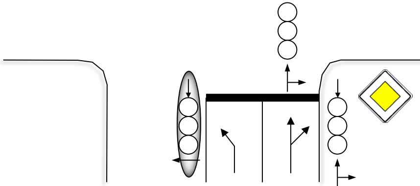
Abbildung 12: Anzahl Signalgeber zwei Fahrstreifen, Haupttrichtung mit Insel (1).
