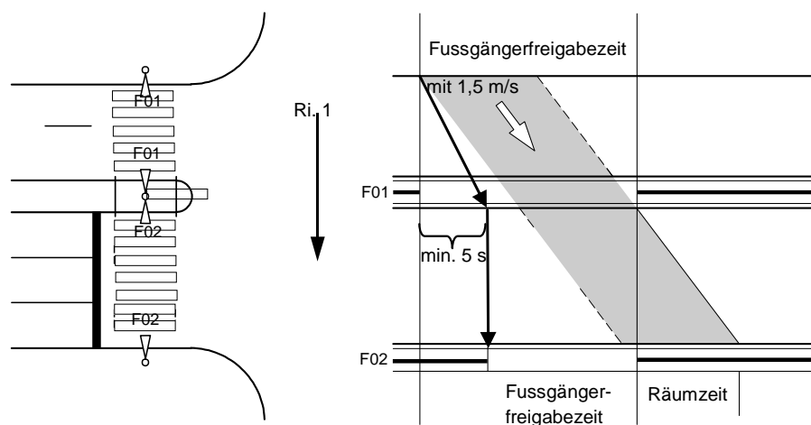
Abbildung 49: Versetzte Gehenzeit (min. 5s, v_{FG} = 1,5 m/s).
