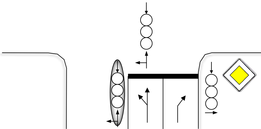
Abbildung 13: Anzahl Signalgeber zwei Fahrstreifen, Haupttrichtung mit Insel (2).
